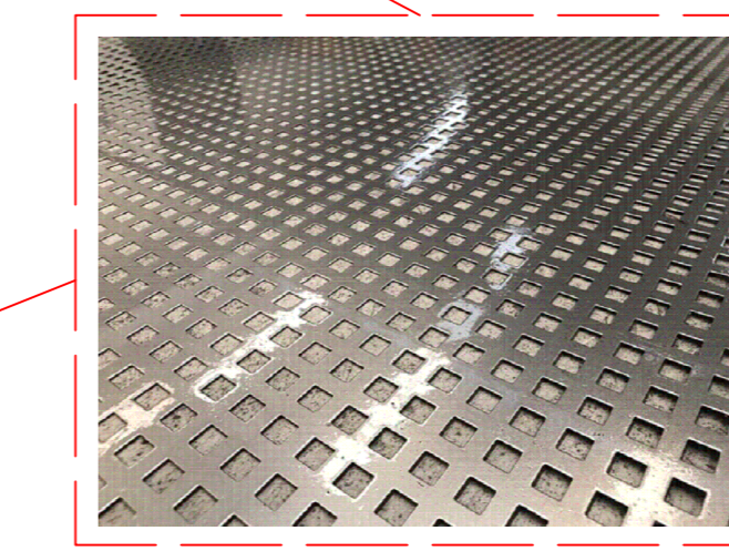
CHAPA GALVANIZADA FURADA PARA FECHAMENTO DOS PÓRTICOS COM ACABAMENTO VERDE BRILHANTE. MODELO QUADRADO DIAGONAL COM FURO 10 mm. ESPESSURA DA CHAPA 1,5 mm.
