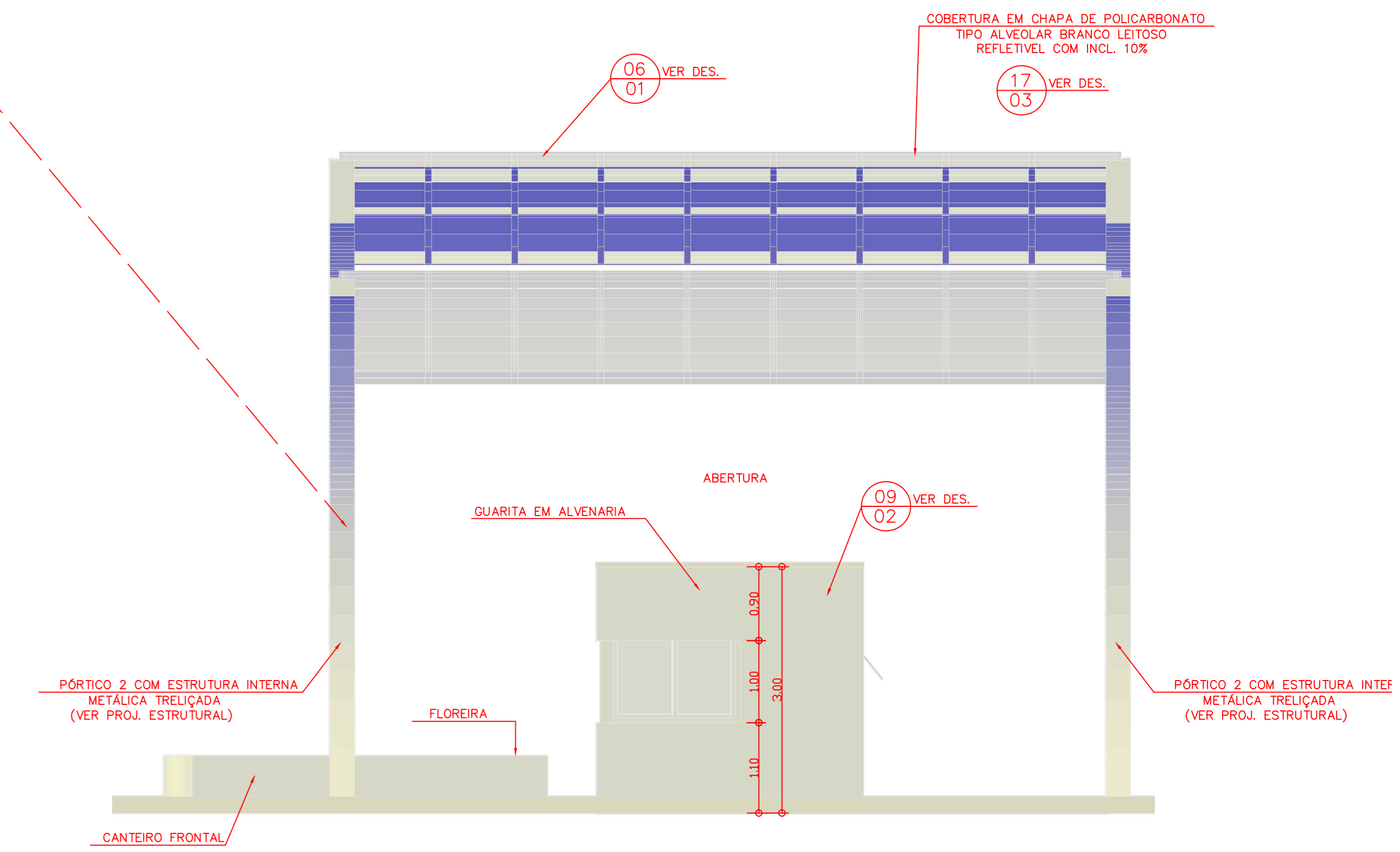
5 VISTA LATERAL DIREITA Esc. 1:50
