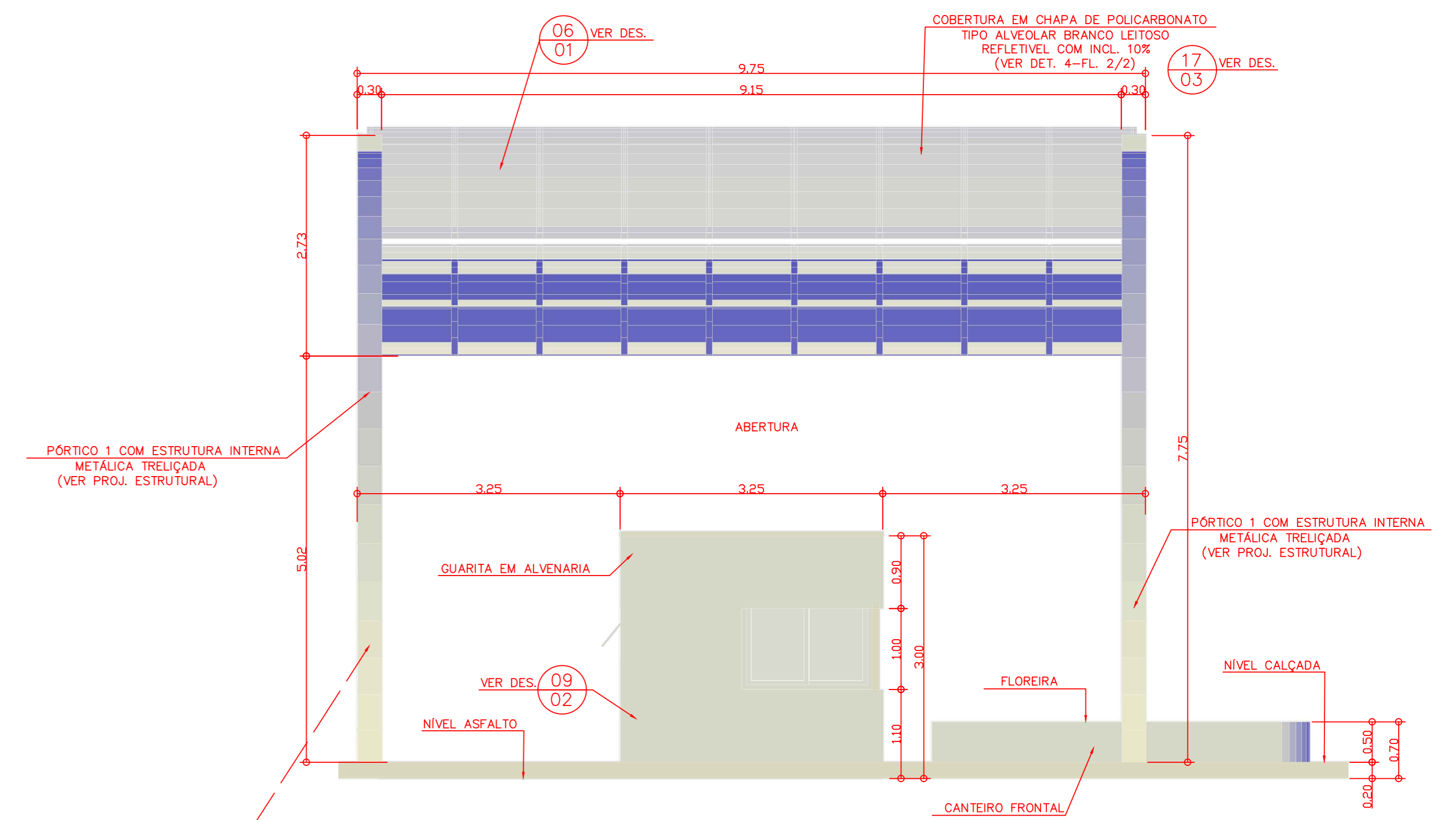
4 VISTA LATERAL ESQUERDA Esc. 1:50
